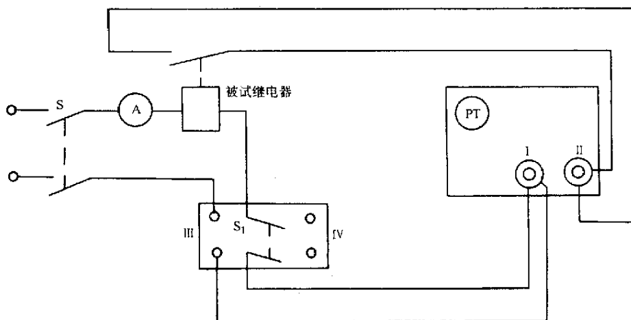
图3 保持值试验接线图
