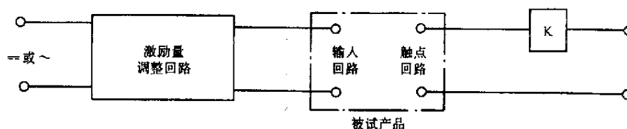
图1 动作值与返回值的试验接线图
