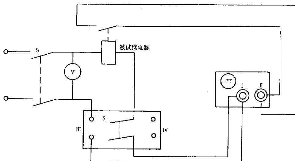
图5 返回时间试验接线图
