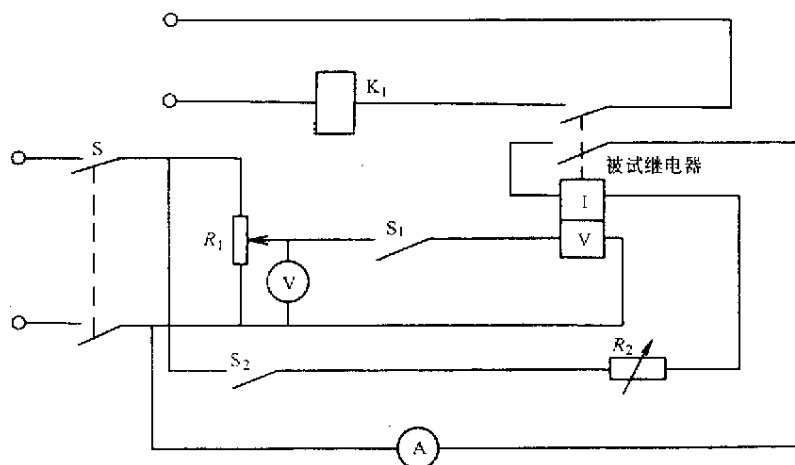
图3 保持值试验接线图
